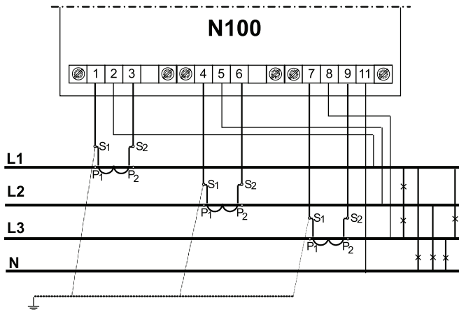
Полукосвенное измерение в 4-проводной сети
