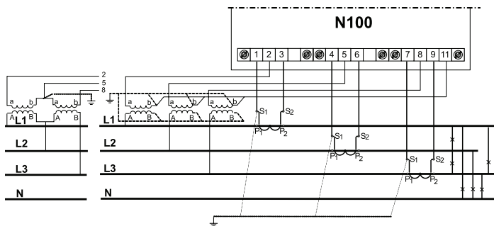
Полукосвенное измерение в 4-проводной сети
