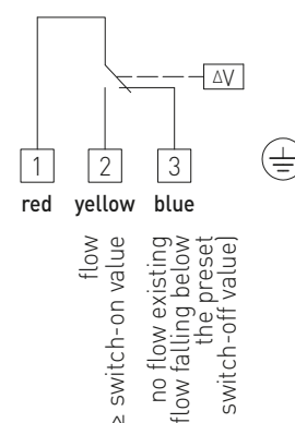
Схема подключения
