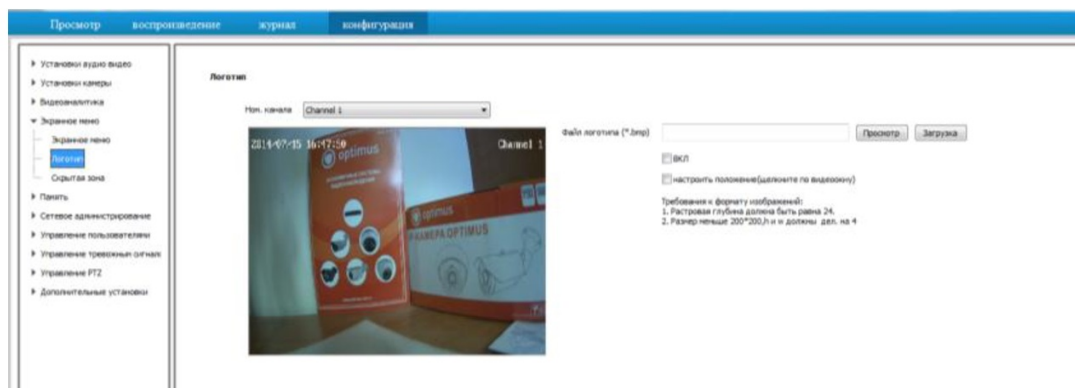
Рис. 4.10.2 Логотип
