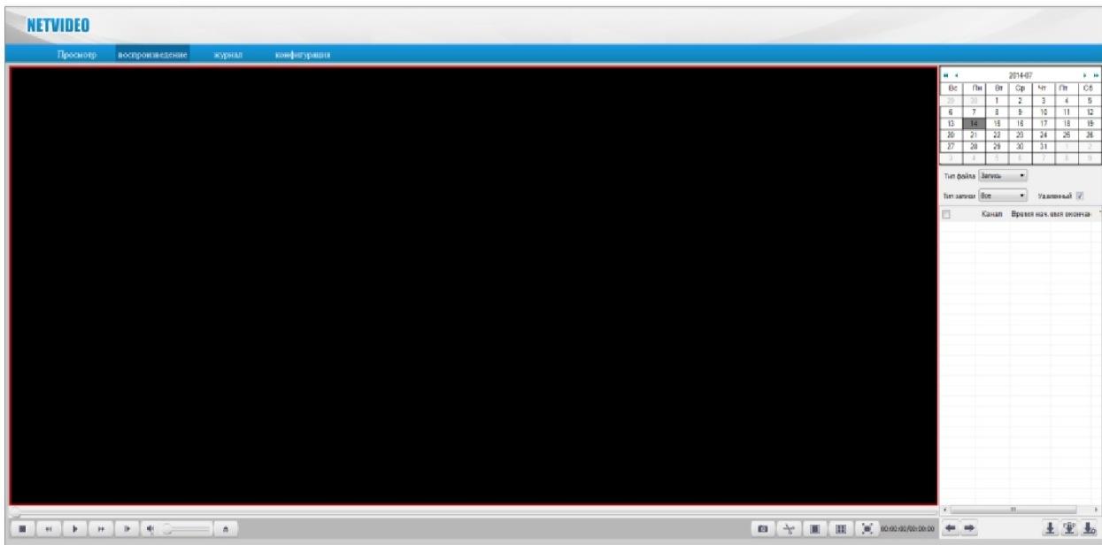
Рис. 4.5.1 Воспроизведение
