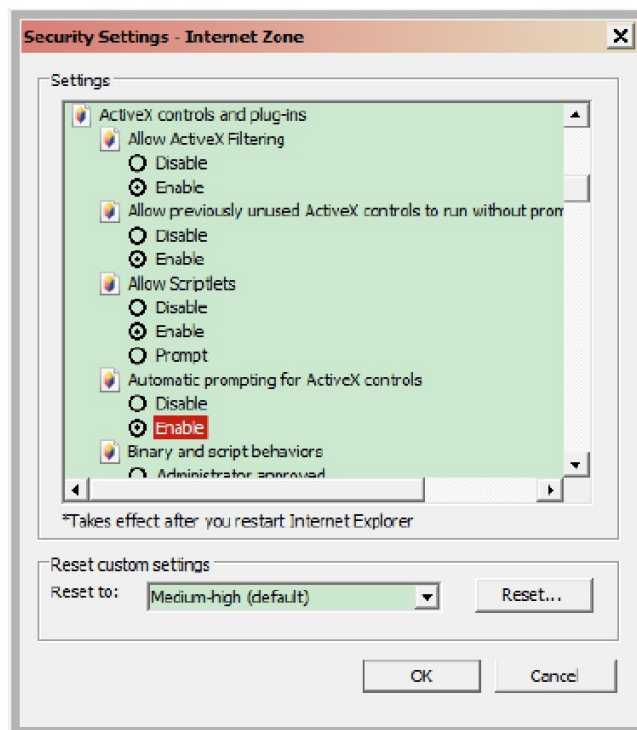
Рис. 5.2.1 Настройки IE
