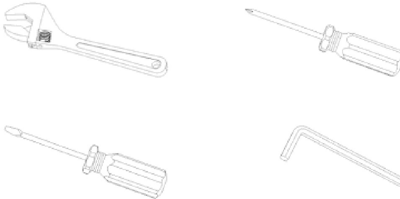
Рис. 3.1.1 Инструменты
