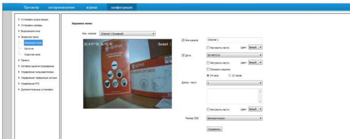
Рис. 4.10.1 Экранное меню
