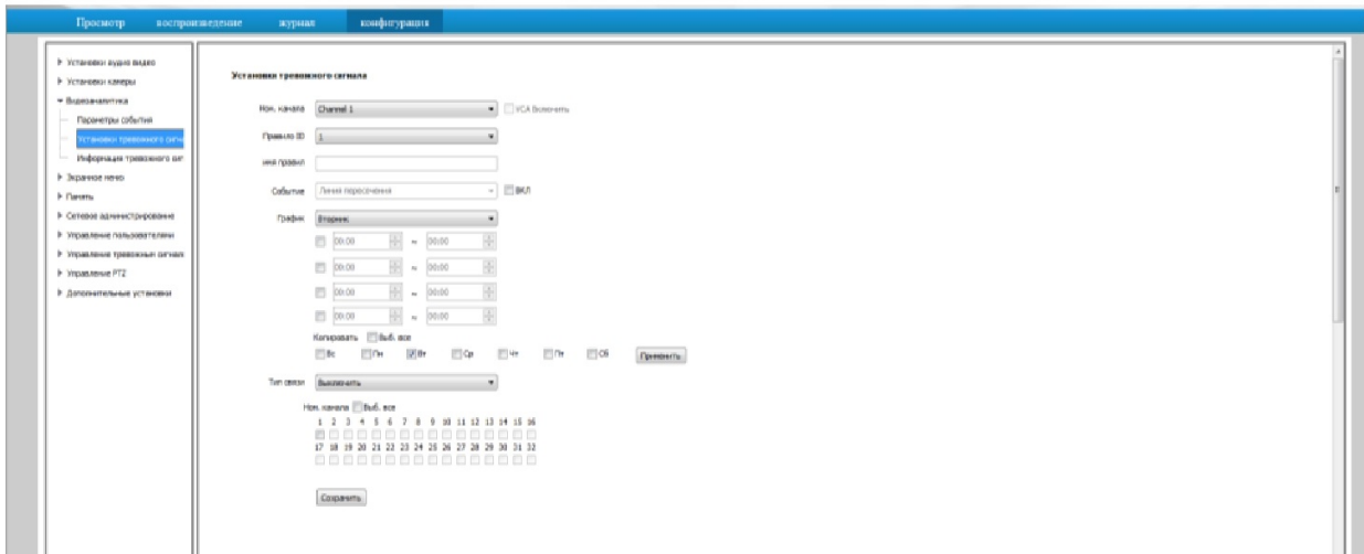
Рис. 4.9.2 Настройки тревоги
