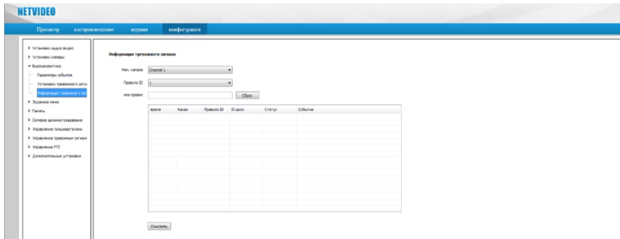
Рис. 4.9.3 Информация тревоги
