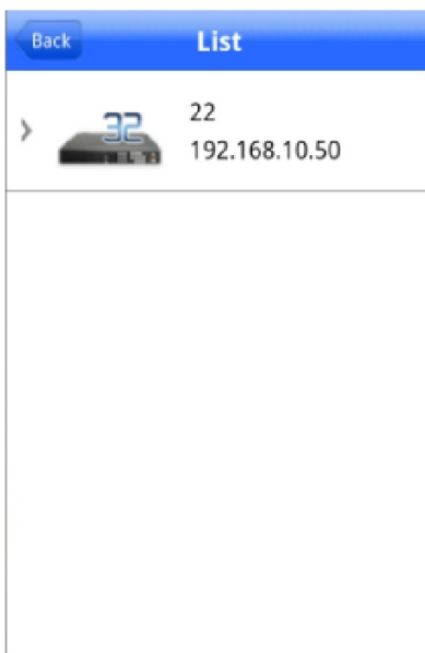
Рис. 4.4. Список устройств
