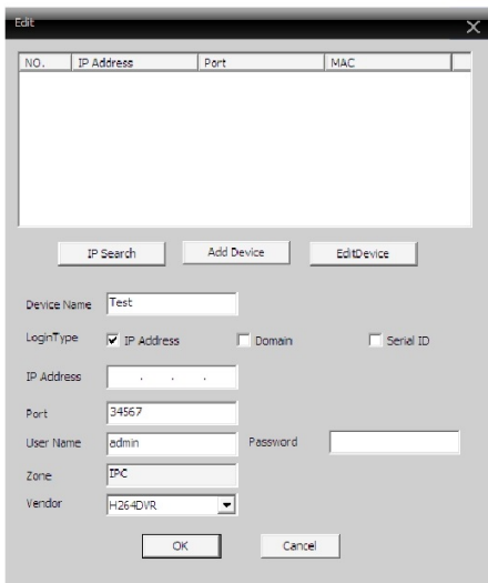
Рис. 2.8 Добавление устройства
