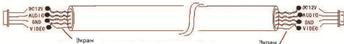
Экранированный сетевой кабель (≤ 40м)
