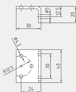
Габаритный чертёж
