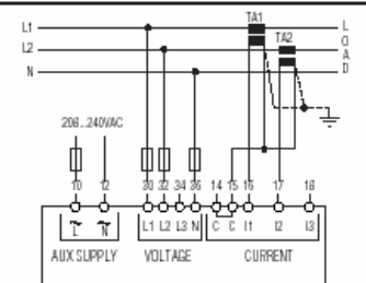
Двухфазное подсоединение Параметр P.03 установлен в 2ph
