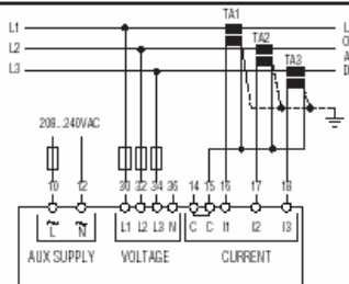
Трёхфазное подсоединение без нейтрали Параметр P.03 установлен в 3ph (по умолчанию)
