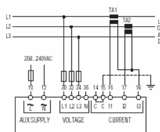
Трёхфазное подсоединение без нейтрали Параметр P.03 установлен в 3ph (по умолчанию) Токовое подсоединение по схеме "Aron"
