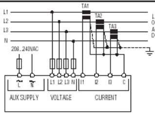
Трёхфазное подсоединение с нейтралью Параметр P.03 установлен в 3ph (по умолчанию)
