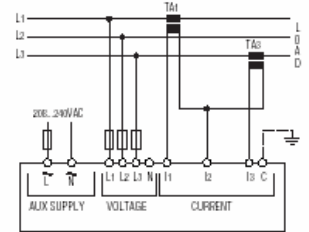
Трёхфазное подсоединение без нейтрали Параметр P.03 установлен в 3ph (по умолчанию) Токовое подсоединение по схеме "Aron"
