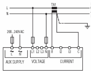
Однофазное подключение Параметр P.03 установлен в 1ph
