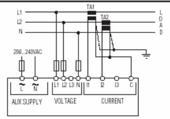
Двухфазное подсоединение Параметр P.03 установлен в 2ph
