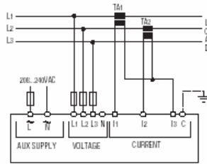
Трёхфазное подсоединение без нейтрали Параметр P.03 установлен в 3ph (по умолчанию) Токовое подсоединение по схеме "Aron"
