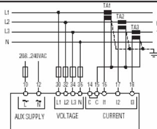
Трёхфазное подсоединение с нейтралью Параметр P.03 установлен в 3ph (по умолчанию)
