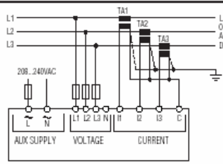
Трёхфазное подсоединение без нейтрали Параметр P.03 установлен в 3ph (по умолчанию)
