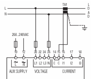
Однофазное подсоединение Параметр P.03 установлен в 1ph
