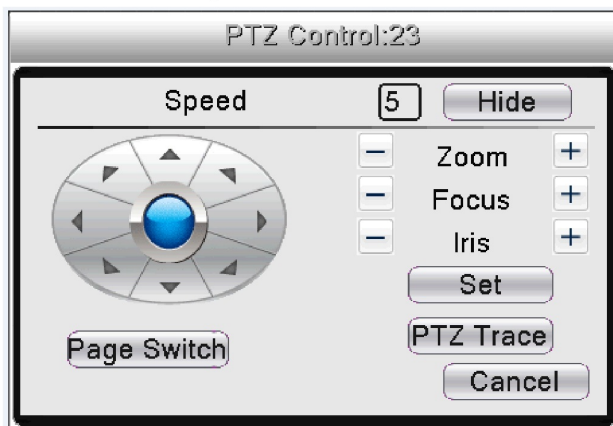
Рис.3.7 Интерфейс управления PTZ функциями
