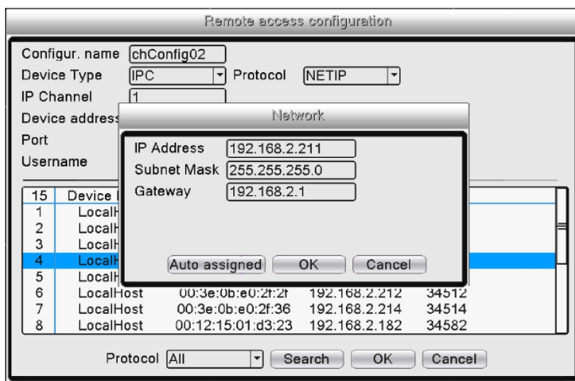
Рис.4.14 Интерфейс настройки IP адреса
