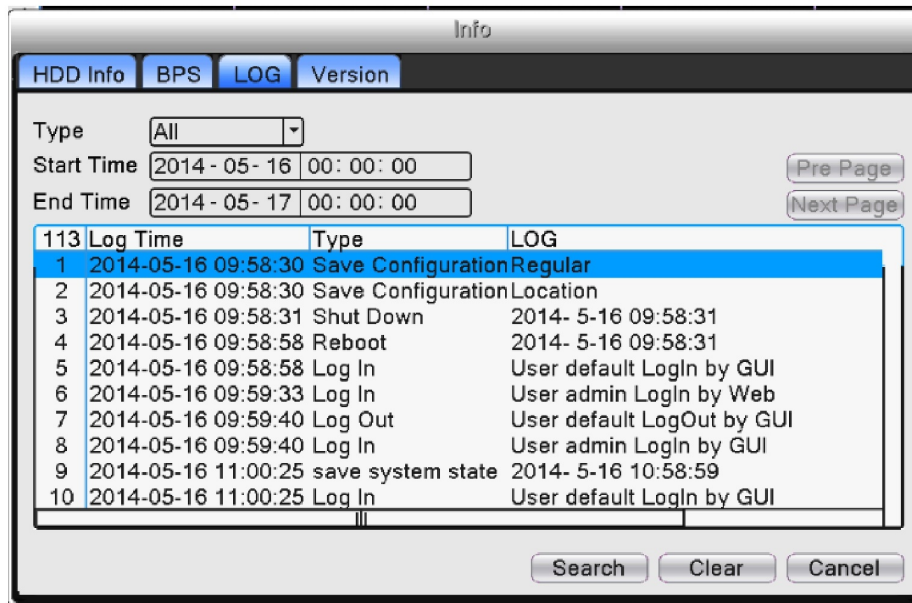
Рис.4.21 Информация системного журнала
