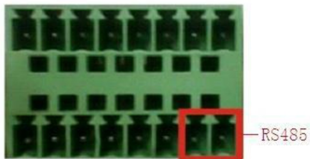
RS485 интерфейс с 8 внешними входами тревог
