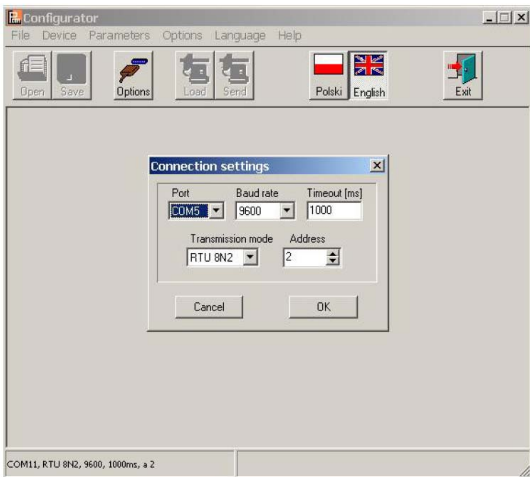
Рис.7. Конфигурирование соединения с прибором N20
