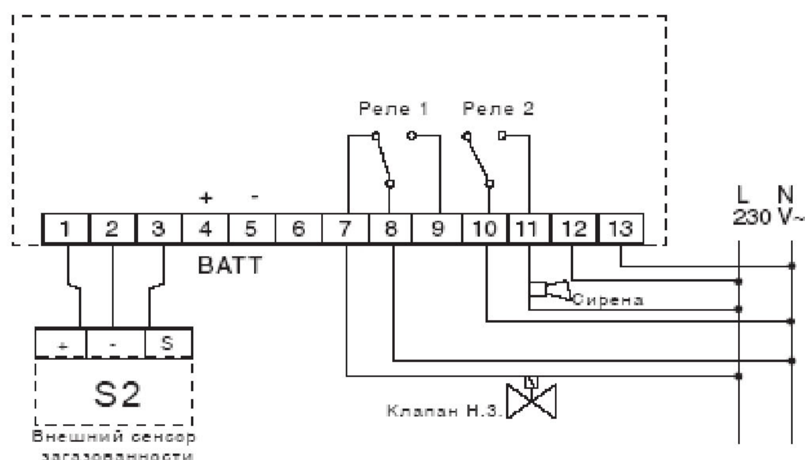
Рис.2 Схема подключения
